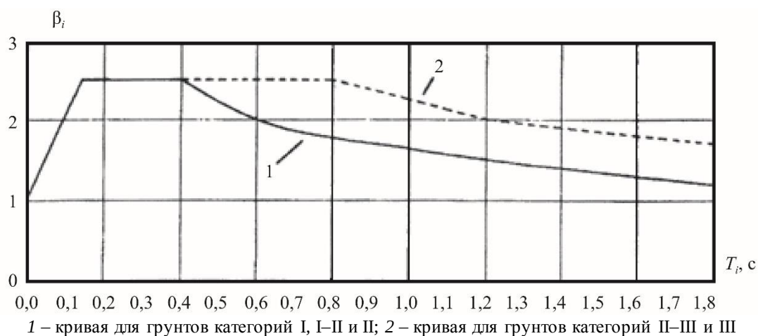
Рисунок 8.1 – Коэффициенты динамичности \beta(T_i)
